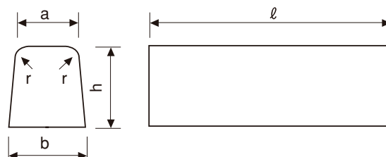
両面歩車道境界ブロック
