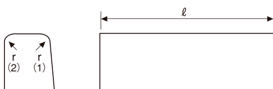
片直両面歩車道境界ブロック
