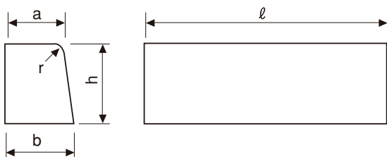
片直両面歩車道境界ブロック
