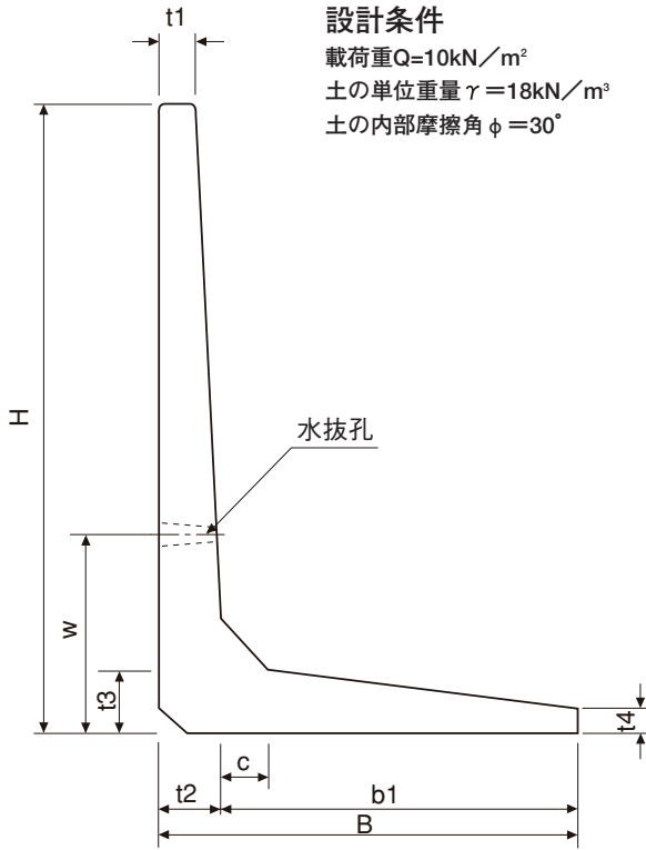
側面図
