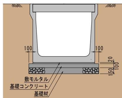
標準断面図
