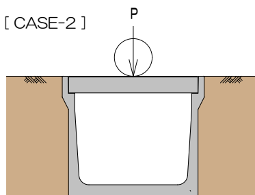
標準断面図
