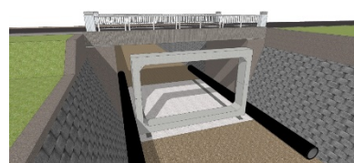
③ 既設橋梁の手前にボックスカルバートをセットし、横引き施工を開始する (横引き施工を繰り返す)
