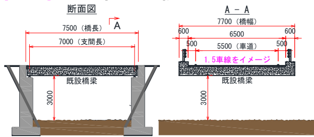
検討モデル（橋長7.5m 橋幅7.7m 桁下3.0m）
