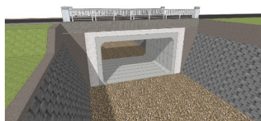
⑤ 既設橋梁との隙間にモルタルを充填し、河床部を埋め戻す
