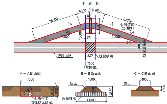
更新（架替え）工事の全体概要図（検討モデル）
