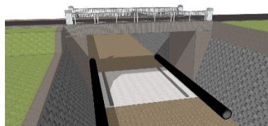
② 仮排水管を設置した後、河床を掘削し基礎コンクリートを打設する
